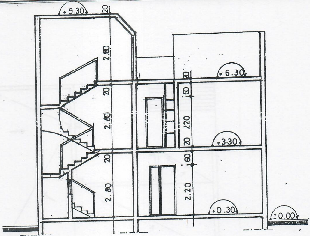
COUPE AA ECH : 1 / 100
