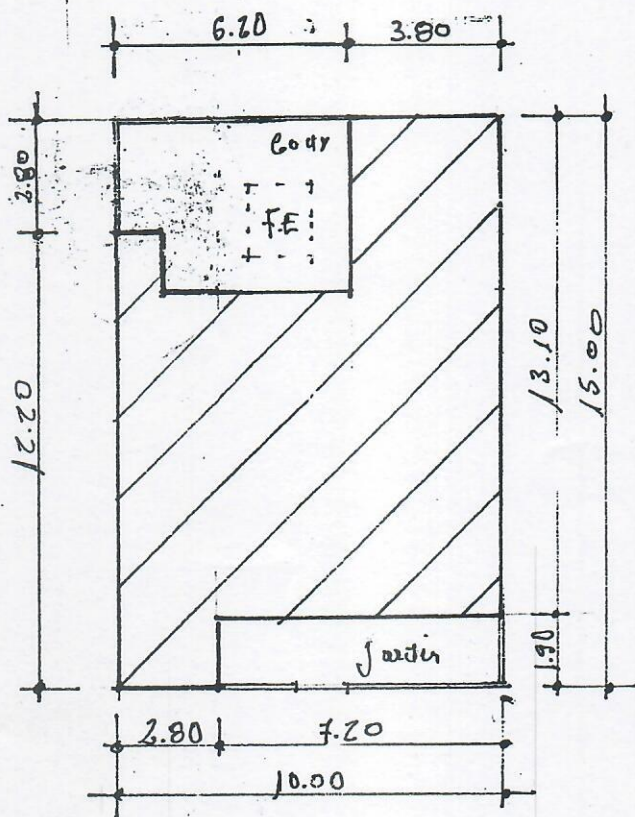
Plan de Masse 1:200 e
